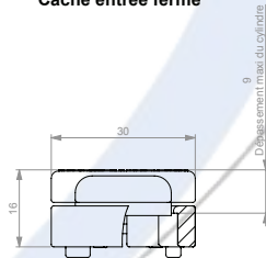
Cache entrée fermé
